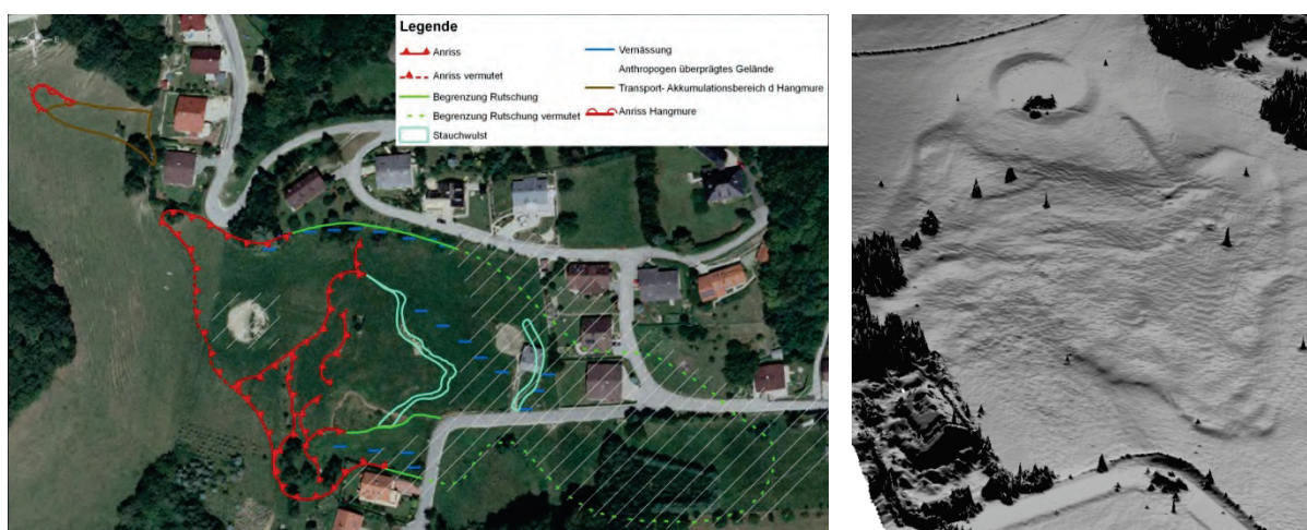
Abb. 10: Rutschung mit Lockermaterialcharakter in stark verwitterten, veränderlich festen Gesteinen der Grestener Klippenzone (JOCHUM et al., 2008); linkes Bild: Kartierung auf Orthofotobasis; rechtes Bild: Laserscan (DOM) des zentralen Rutschungsbereichs.
